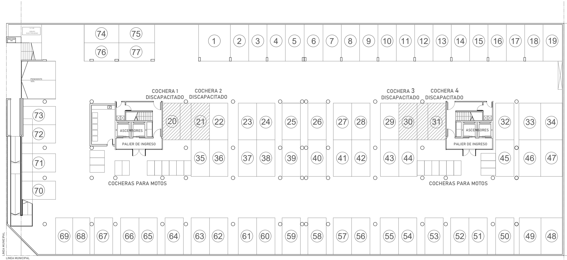
PLANTA COCHERAS
